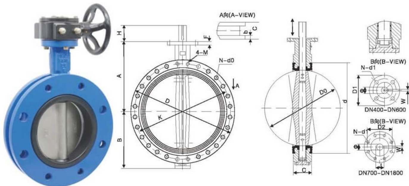
主要连接尺寸 Main connection dimensions
