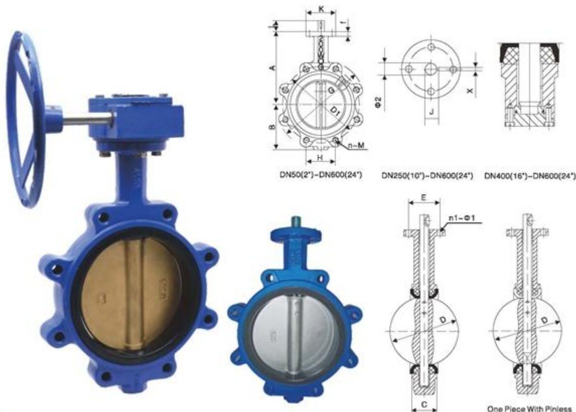
主要连接尺寸 Main connection dimensions
